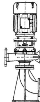
דגם ACMV משאבת מונובלוק במבנה אנכי
