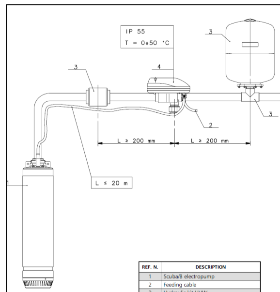
מתקן הגברת לחץ עם משאבה טובולה מסדרה SC ומשנה תדרים הידרואר WATER COOLED
